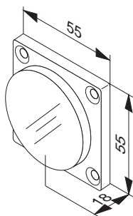
GT 50 R 5 Contre-plaque à ressort pour GT 50 R xxx Spring loaded counterplate for GT 50 R xxx
