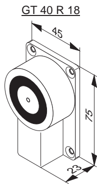
GT 40 R 18 Ventouse magnétique pour porte, Force de maintien : 300 N Magnetic clamp for fire door, hold-on power: 300 N
