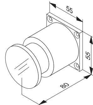
GT 50 R 7 Boulon d'ancrage télescopique avec contre-plaque pour GT 50 R xxx Telescopic anchor with counterplate for GT 50 R xxx
