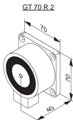
Ventouse magnétique pour porte, Force de maintien : 1372 N Magnetic clamp for fire door, hold-on power 1372 N
