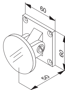
GT 50 R 6 Contre-plaque à ressort pour GT 50 R xxx, Plage de pivotement \pm 60^\circ Spring loaded counterplate for GT 50 R xxx, swivelling range \pm 60^\circ
