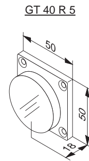
GT 40 R 5 Contre-plaque à ressort pour GT 40 R 18 Spring loaded counterplate for GT 40 R 18
